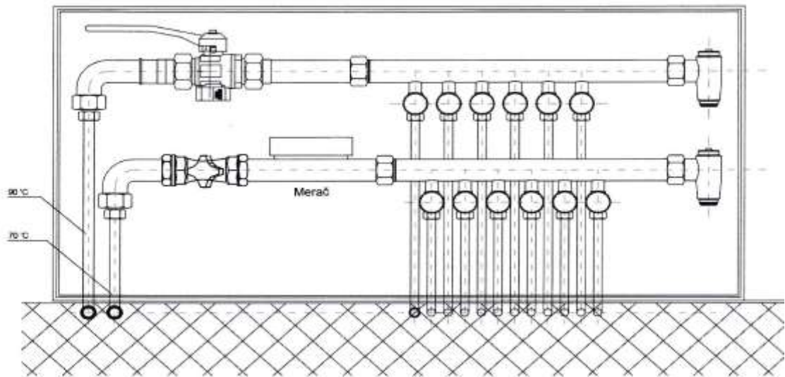
Šema kasete za razvod cevi u stanu
